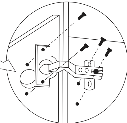
Detalhe da Colocação das Dobradiças
